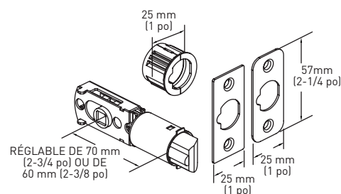
LOQUET D'ENTRÉE 6-EN-1 RÉGLABLE
