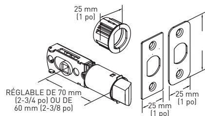
LOQUET 6-EN-1 VERROUILLABLE /NON VERROUILLABLE
